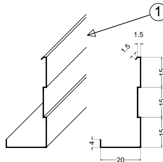
Cenefa-chapa galv. N°22 FRENTE IDEM CANALETA 30ml
