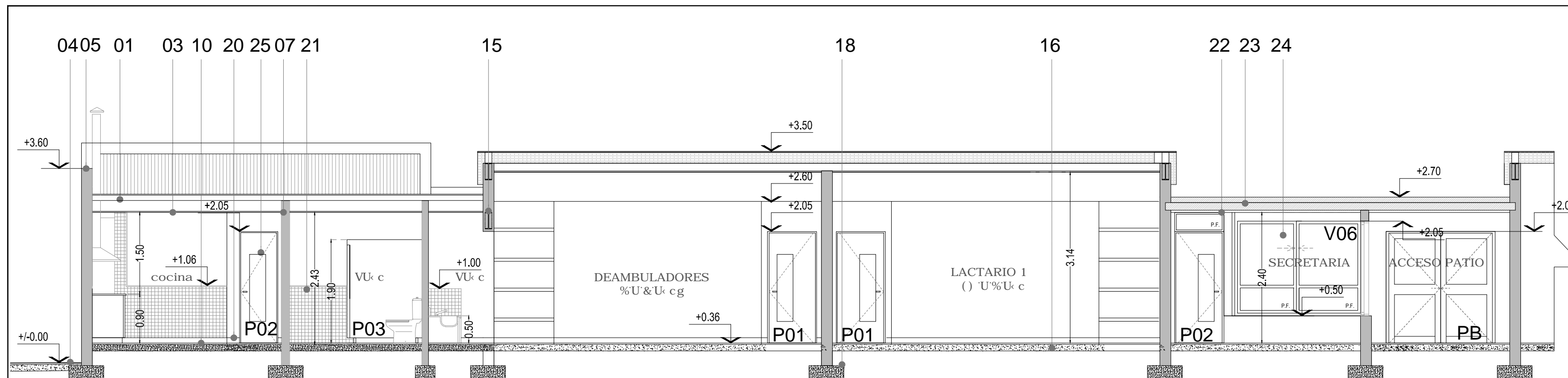
CORTE 2-2
